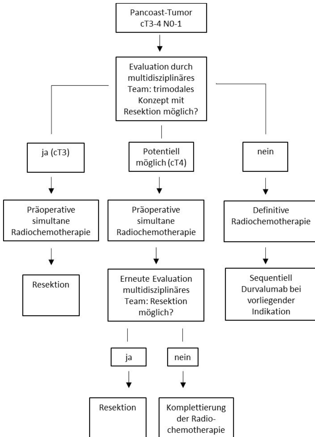
Abbildung 13: Algorithmus Pancoast-Tumor
